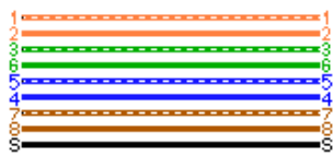
Mapa de hilos: T568B
